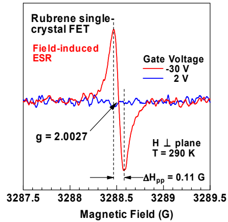
図 4 ルブレ単結晶 FET のゲート電圧誘起 ESR 信号。実線はゲート電圧が -30 V、点線はゲート電圧が 2 V の信号を示す。
