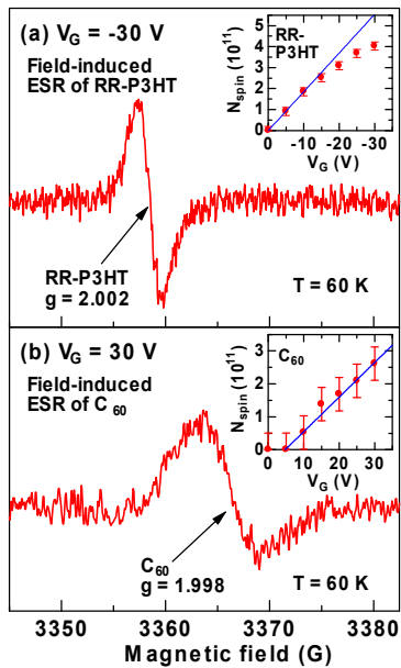
図 3 (a) RR-P3HT に起因した RR-P3HT- C_{60} 複合体 MIS ダイオードのゲート電圧誘起 ESR 信号。(b) C_{60} に起因した RR-P3HT- C_{60} 複合体 MIS ダイオードのゲート電圧誘起 ESR 信号。挿入図：ゲート電圧誘起されたスピン数のゲート電圧依存性。
