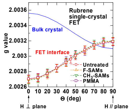
図 5 ルブレ単結晶 FET のゲート電圧誘起 ESR 信号の g 値の角度依存性。空丸 ( \circ ) は界面未処理 FET の結果を示す。上三角 ( \triangle )、下三角 ( \nabla )、空四角 ( \square ) のデータは、それぞれ F-SAMs、 \text{CH}_3 -SAMs、PMMA による界面修飾 FET の結果を示す。 \theta は外部磁場と基板のなす角度を示す。測定温度は 290 K。実線はバルク結晶で予想される g 値の角度依存性。
