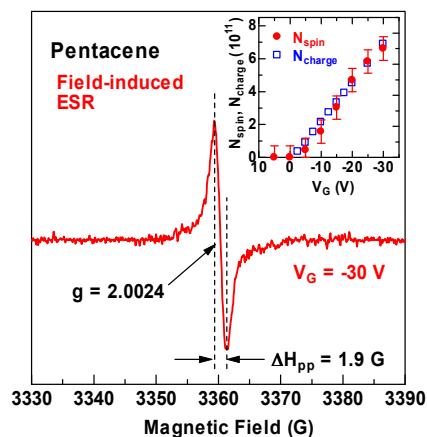
図 2 ペンタセン FET のゲート電圧誘起 ESR 信号。挿入図：ゲート電圧誘起スピン数のゲート電圧依存性 (実丸) とゲート電圧誘起電荷数のゲート電圧依存性 (空四角)。
