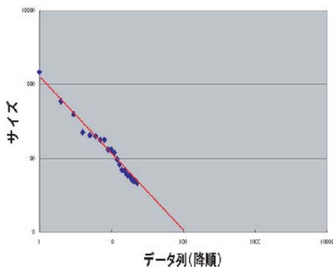
図 11 竜安寺の石庭に対してすべての石と群のサイズを Hausdorff 距離で測定しそのサイズデータを降順に並べて、両対数を求めて傾きを調べると-1.04 になる Fig.11 we with Hausdorff distance method to measure all the stone's and group's size of Ry-ouan-ji garden, then size of the data to be arranged in descending order of the double logarithmic coordinate .the slope is -1.04
