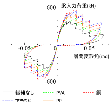
図10 柱梁接合部繊維種類の比較
