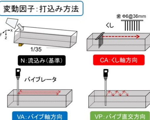
図 3 繊維の配向性を制御する打込み
