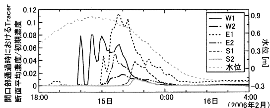
図-12 Tracer 断面平均濃度時系列
