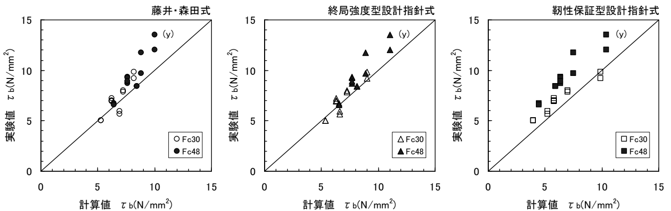
(y):主筋降伏 図9 付着強度の実験値と修正式による計算値との比較
