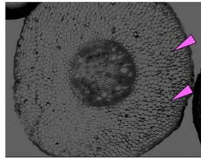
図2 光屈性刺激にともなうリグニンの蓄積 (トウモロコシ芽生え、右側から刺激を与えた)
