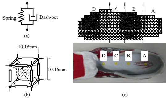
図 3-1. シューズのモデル化 (a)トラス要素, (b)立体的トラスモデル, (c)ソールモデル
