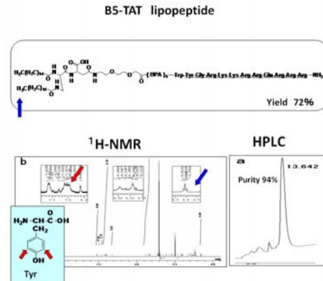
【図1 Lipopeptide の合成と収率検討】
