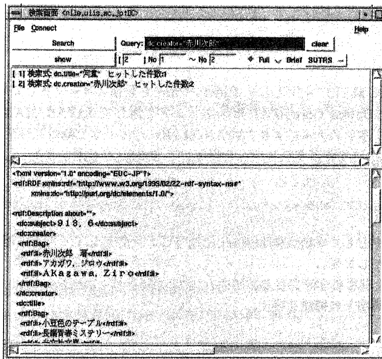
図 2: 検索例
