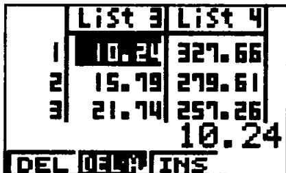
図3 入力画面
