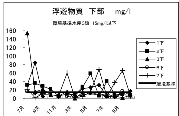
図 10. 各調査地点下部の浮遊物質季節変化
